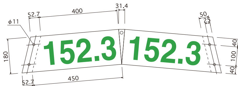
展開図 Scale1/10
