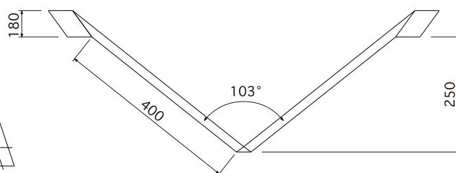
平面図 Scale1/10
