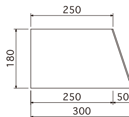
側面図 Scale1/10
